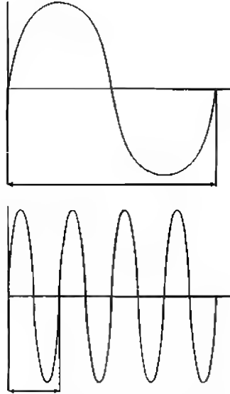
المشكل (٦ - ٣) موجات ساين: أطوال الموجات موضحة بالأسهم
